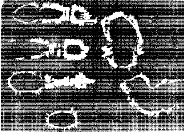
شكل ( ١٠ هـ ) الصورة توضح بدا بشرية بالتصوير الكيرليانى ، ومن كل اصبح تنطلق شحنة مختلفة تبدو على هيئة هالة على الفيلم الحساس .
